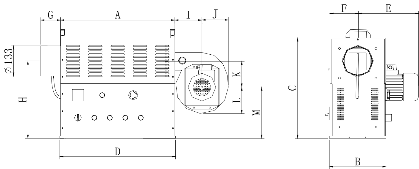
尺寸图
