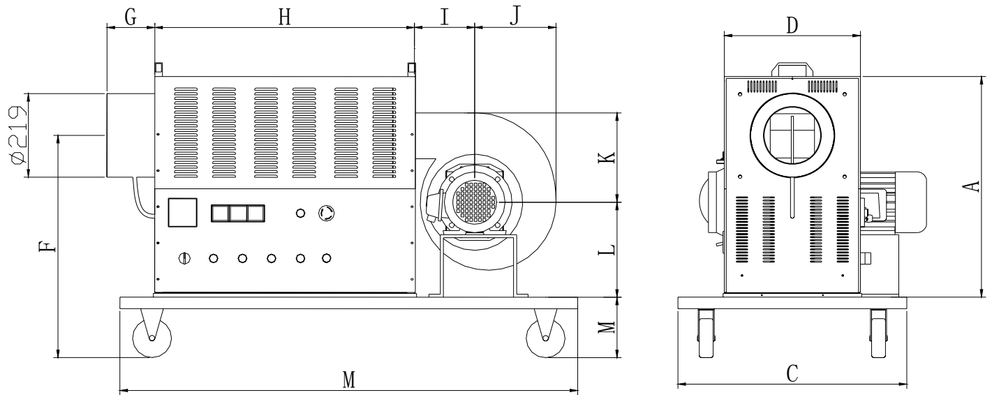
尺寸图
