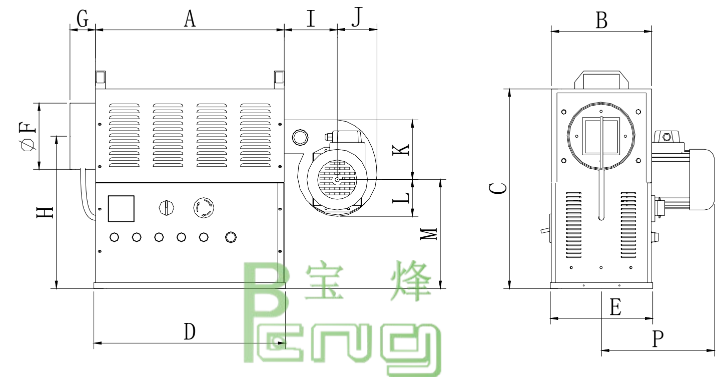
尺寸图
