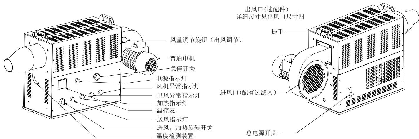
功能指示图
